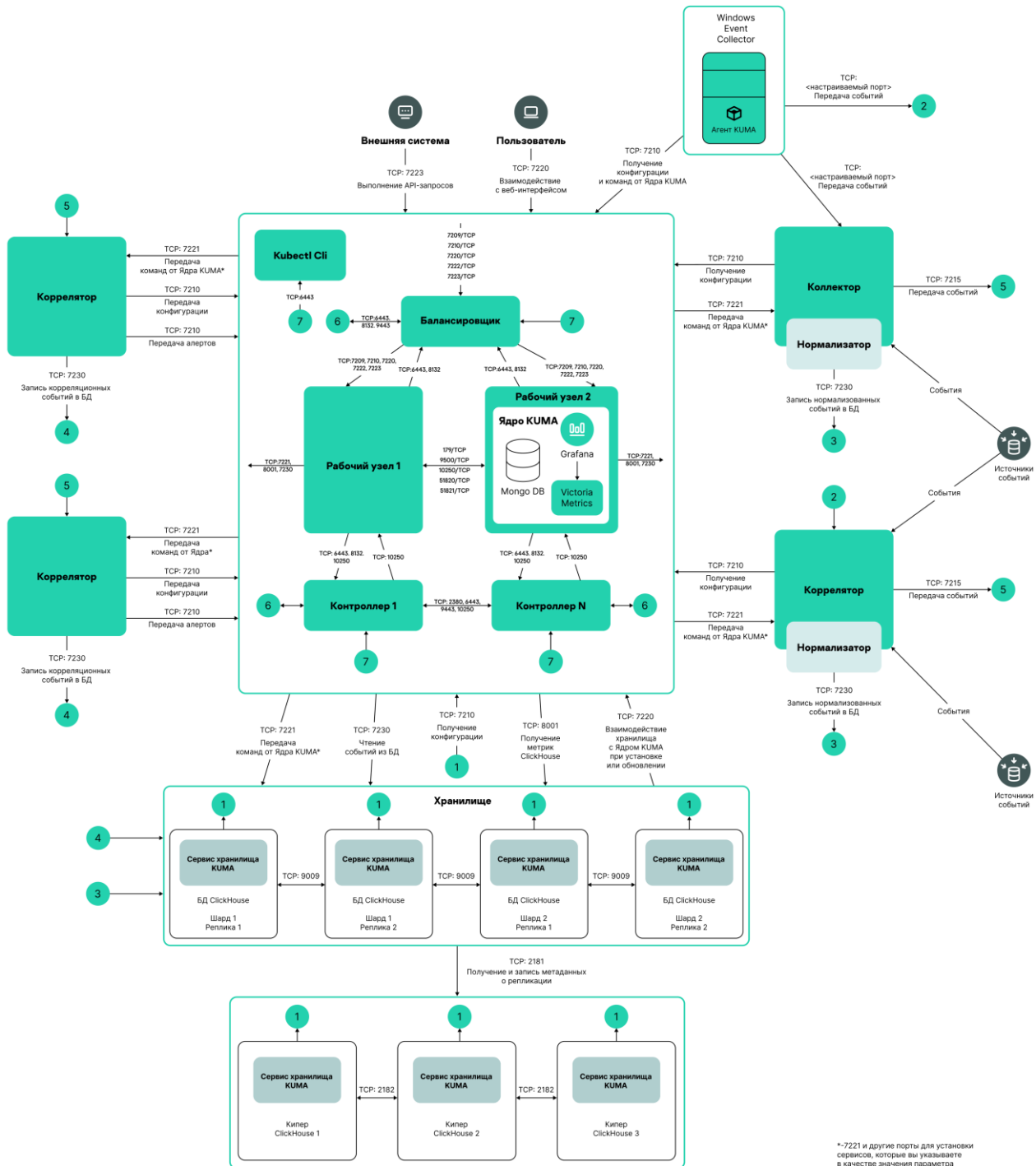
Рисунок 5. Распределенная установка в отказоустойчивой конфигурации
