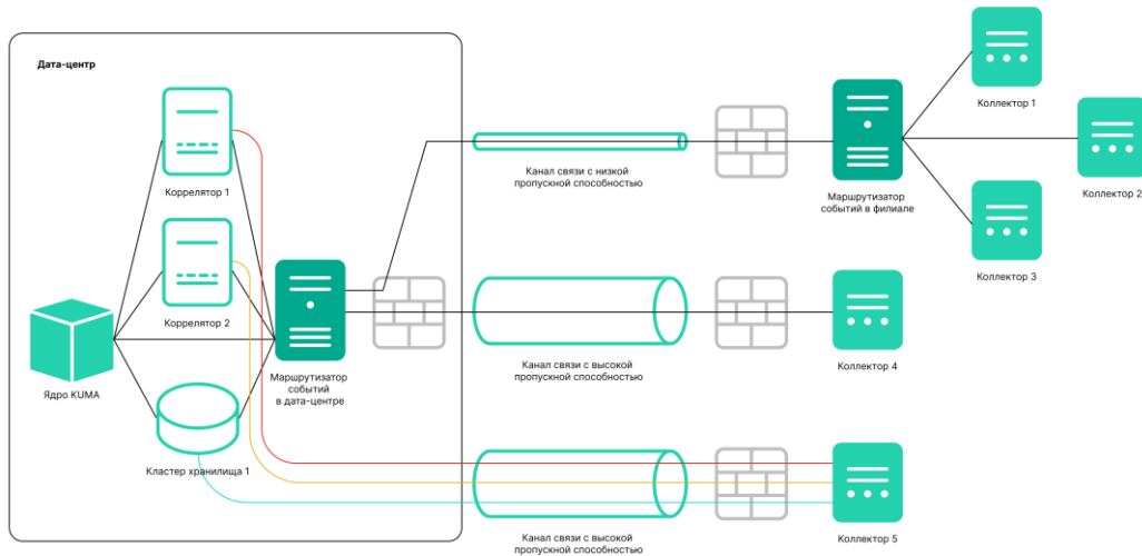
Рисунок 1. Схема отправки событий с использованием маршрутизатора событий и без использования маршрутизатора
