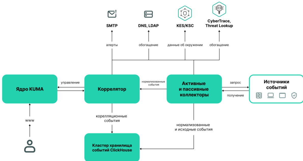
Рисунок 2. Архитектура KUMA
