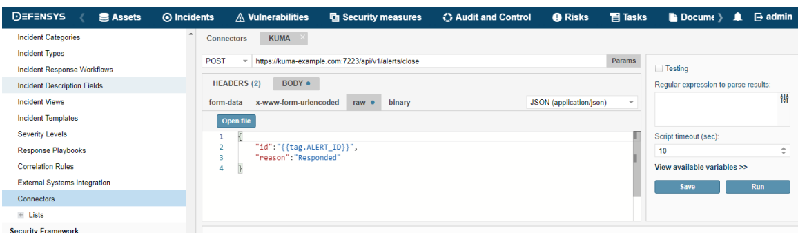
Рисунок 25. Тело API-запроса
