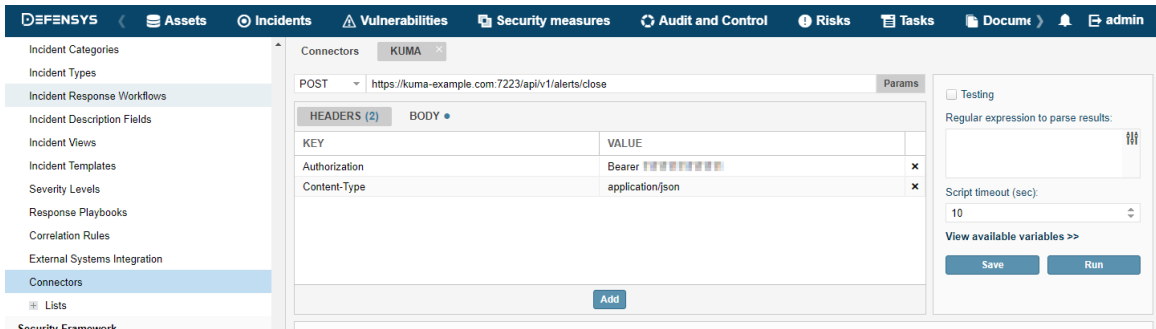
Рисунок 24. Заголовок API-запроса
